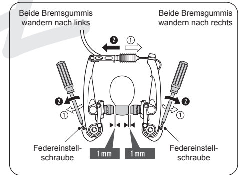
Einstellen der Bremsen an der Felge
